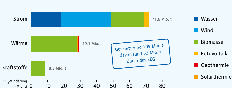
Vermiedene CO 2 -Emissionen durch die Nutzung erneuerbarer Energien in Deutschland im Jahr 2008
